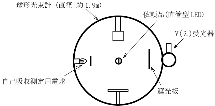
備考図 1 測定時の配置
